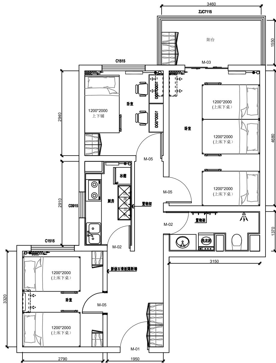
平面布置图
